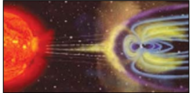
تأثير المجال المغناطيسي أو حزام فان ألين الذي مصدره الحديد على الرياح الشمسية
